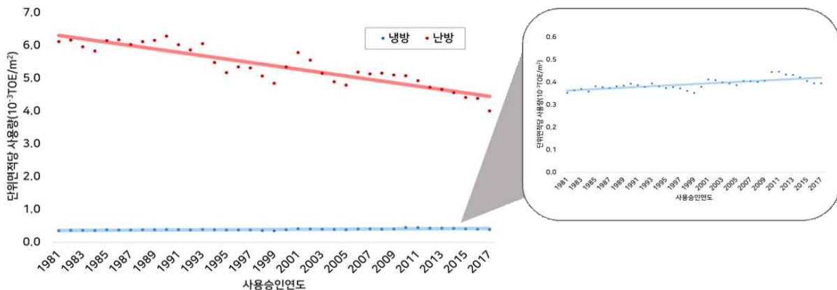
<사용승인 연도별 주거용건물 단위면적당 냉난방 에너지사용량>
