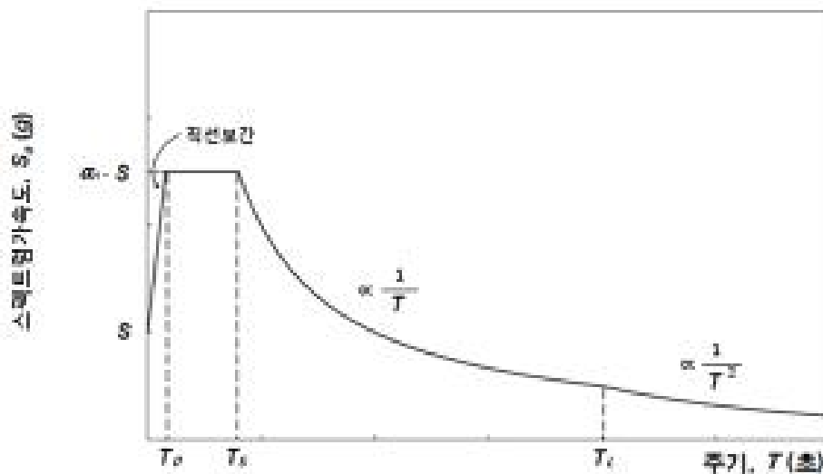
그림 4.2-1 가속도표준설계응답스펙트럼 (암반지반)
