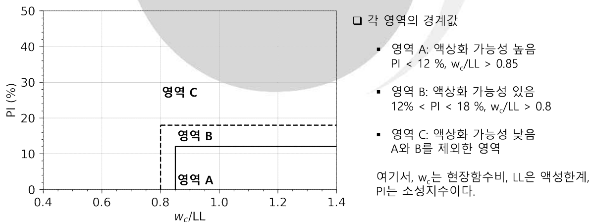
그림 4.7-1 소성지수 기반의 액상화 가능 범위
